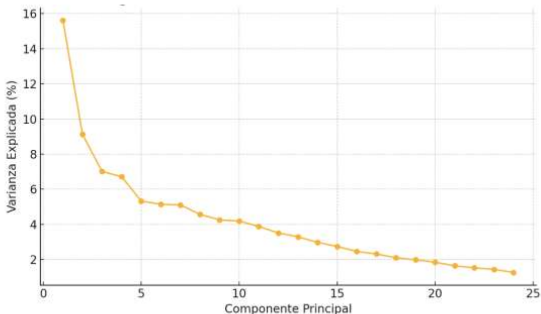
Figura 1. Grafico de sedimentación (ACP).
