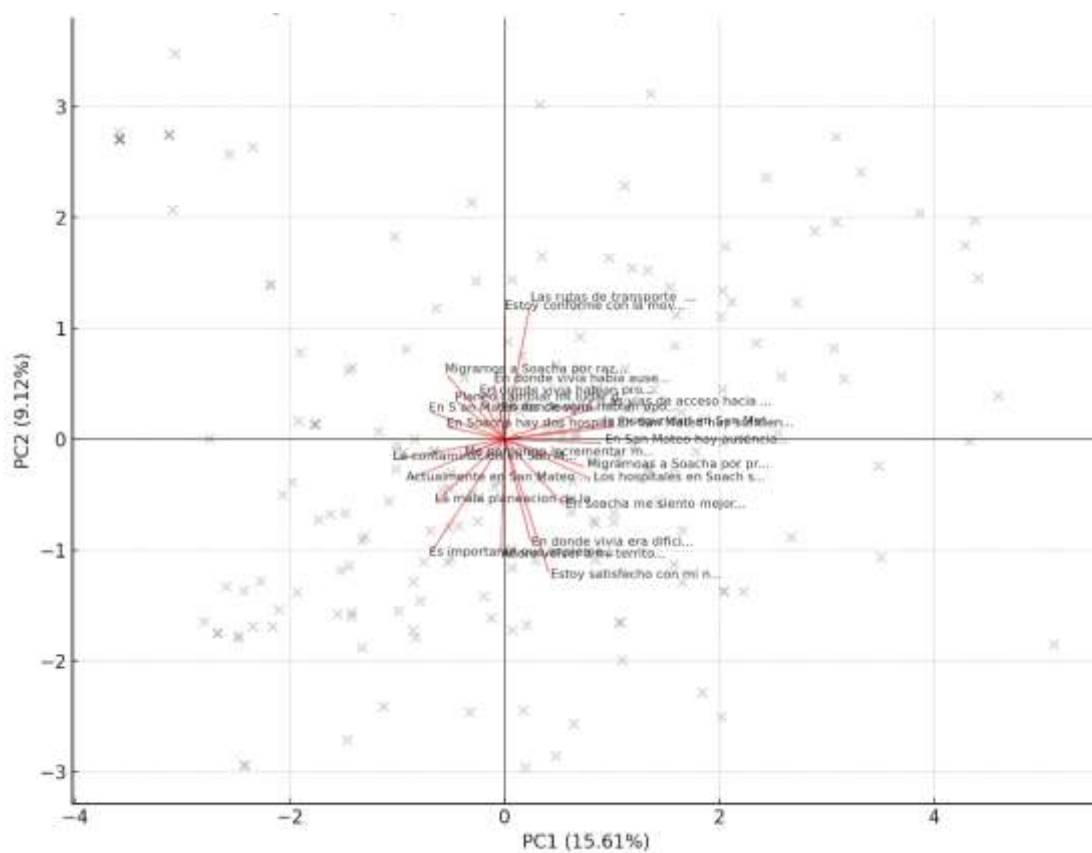
Figura 2. Biplot del Análisis de Componentes Principales (ACP).
